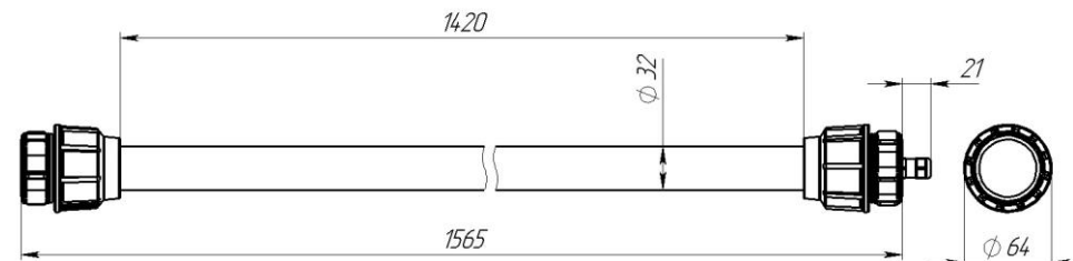
Рисунок 2 Светильник «L-line».
